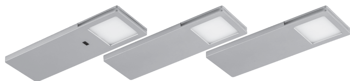
AL8101 Размеры, мм 2,5Wx3 190x66x8 (размер одного светильника) Комплект из 3-х светильников и блока питания 12V Оснащен инфракрасным датчиком движения руки Соединительный провод 1,9 м Сетевой шнур 1,5 м
